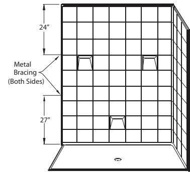
PERSPECTIVE VIEW - N.T.S.
